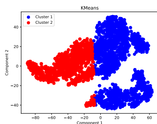
図 5.22 8 層目でのクラスタリング
