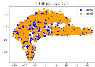
図 5.32 4 層目での出力
