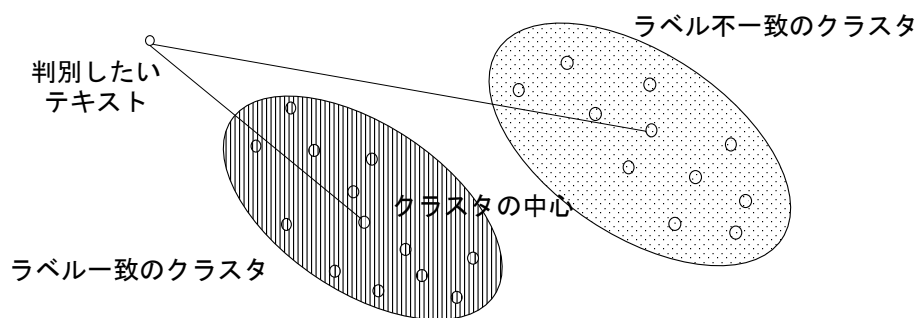
図 4.4 ラベルの一致・不一致の判別の図
